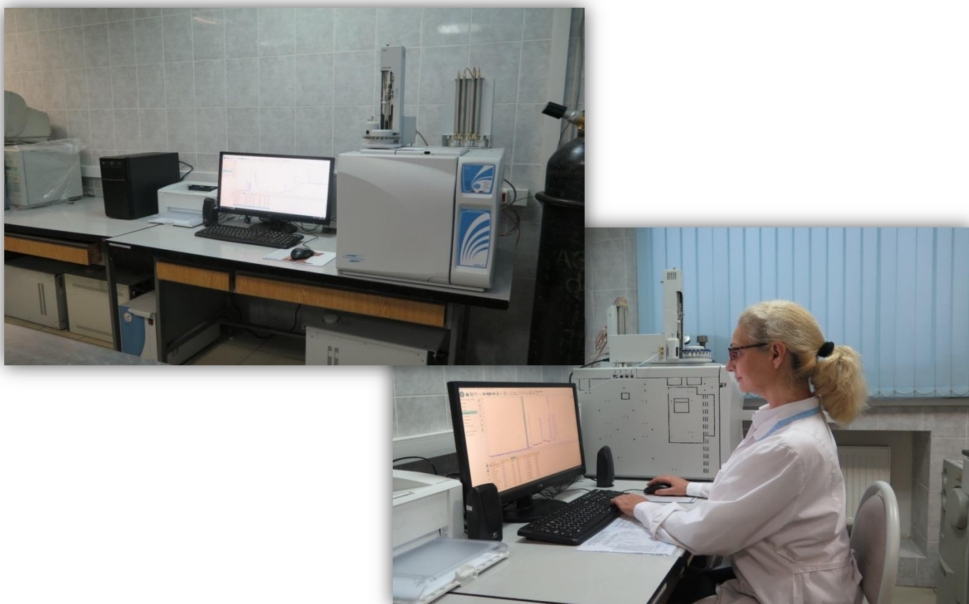
Аппаратно-программный комплекс на базе хроматографа «Хроматэк-Кристалл 5000»
